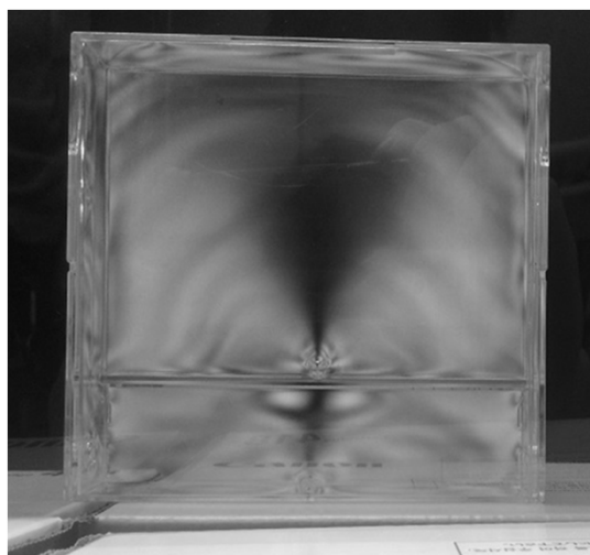
光弾性で見る力の分布
